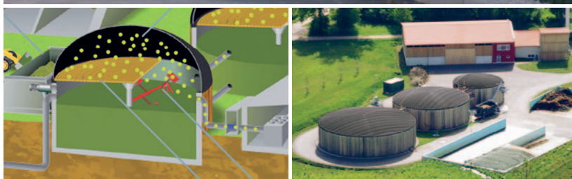
Oben: Ansicht des Fermenters und Nachfermenters; unten links: Funktionsschema der Biogasanlage; unten rechts: fertiggestellte Biogasanlage
